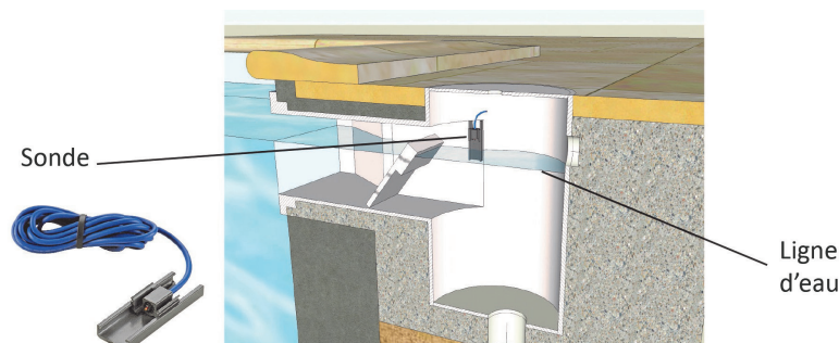
Emplacement de la sonde du NIVEAU dans un skimmer
